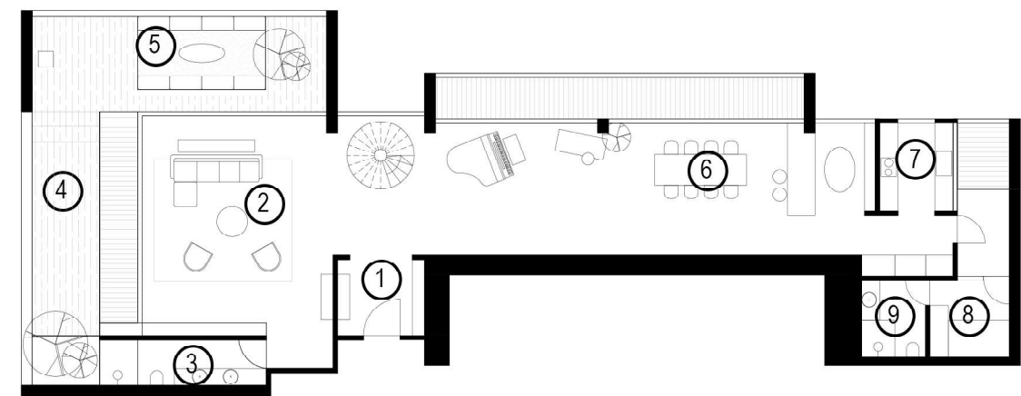
MẶT BẰNG TẦNG 1
